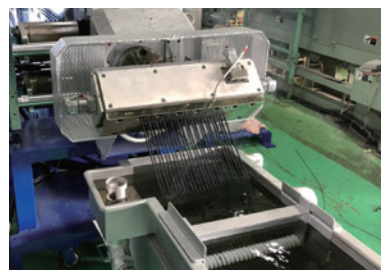
押出機でリサイクルペレットへ
